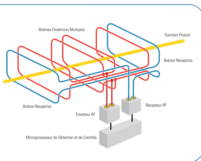
Architecture de la détection à multi spires de l'APEX 500
